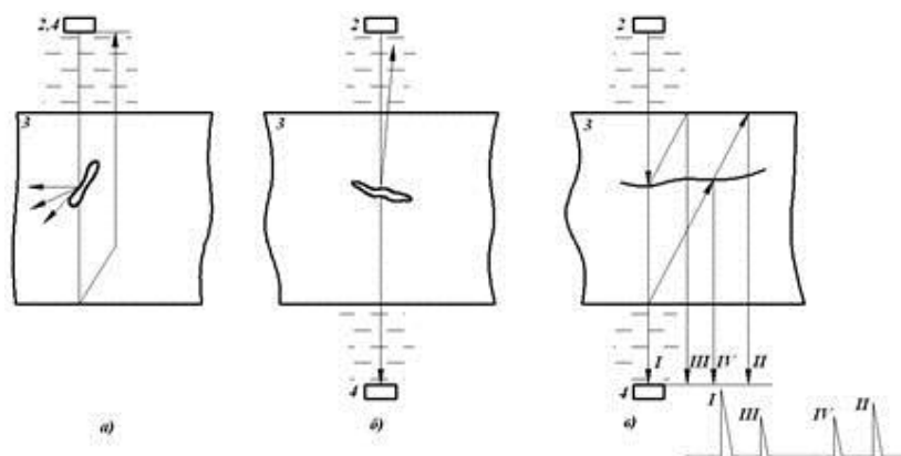
Рис. 1. Комбинированные методы, использующие прохождение и отражение: а - зеркально-теневой; б – эхо - теневой; в – эхо - сквозной; 2 - излучатель; 4 - приемник; 3 - объект контроля
