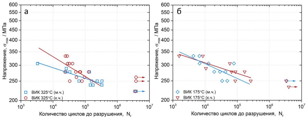
Рис. 1. Зависимости количества циклов до разрушения сплава 1570С с крупными (о, \Delta ) и мелкими ( \square , \diamond ) частицами после 1-го (а) и 3-го (б) этапов ВИК от максимальных напряжений в цикле.
