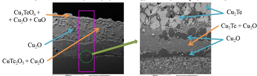
Рис. 4. Распределение фаз в продукте коррозии на основании РФА и СЭМ-РСМА.
