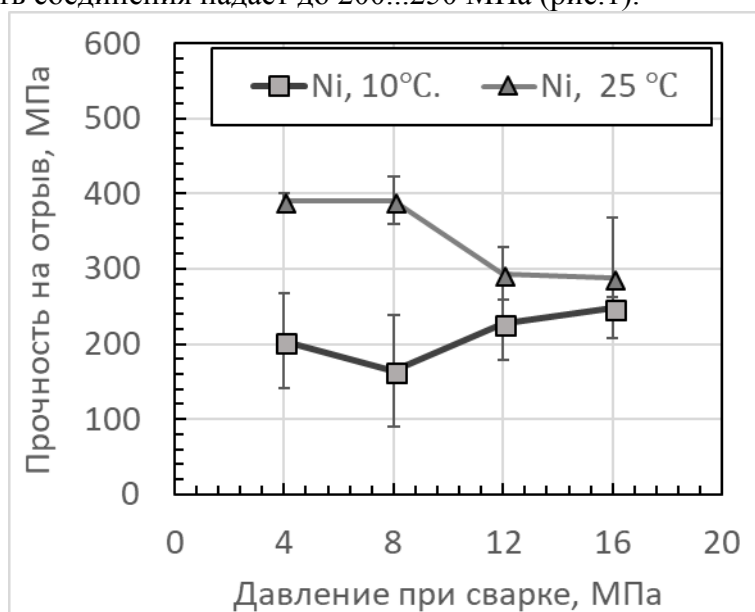
Рис. 1. Влияние сварочного давления на прочность соединения титанового сплава ПТ3В и нержавеющей стали 12Х18Н10Т через прослойку из никеля.
