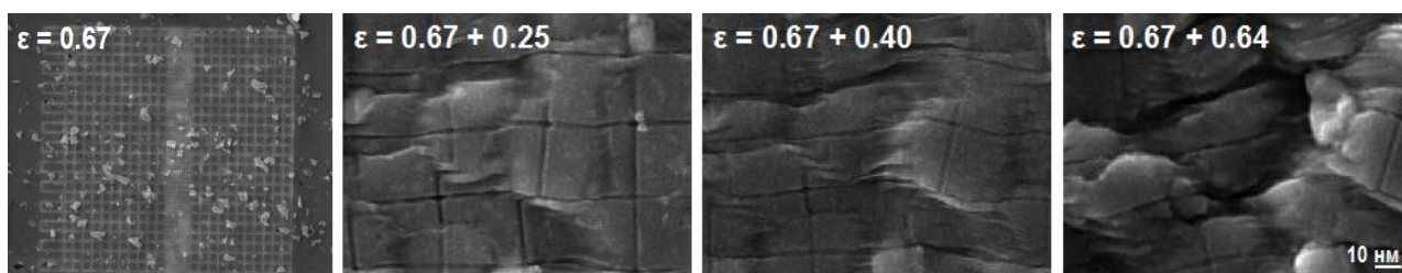
Рис. 1. Изменение поверхности образца с маркерными сетками в процессе последовательной деформации сплава (2) со скоростью 2 \cdot 10^{-3} \text{ c}^{-1} при температуре 480 °С
