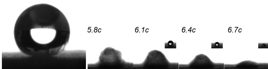
Рис. 2. Капля воды на поверхности графенового нанокompозита в режиме Лейденфроста (а), нарушение стабильности левитации (б)
