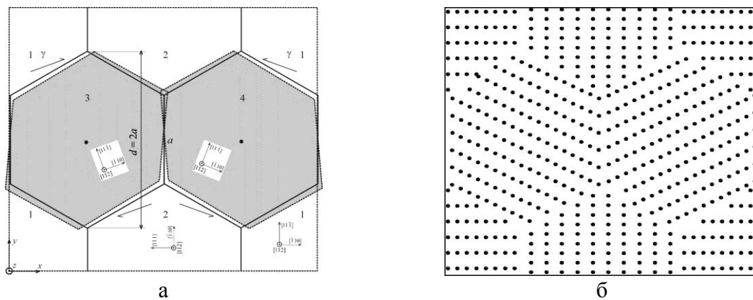
Рис. 1. Схема метода построения расчетной ячейки г.ц.к. нанокристалла с осью колонны [112] с неравновесными ГЗ (а) и исходная структура нанокристалла с размером зерен d = 5 нм и деформацией сдвига \gamma = 0.15 зерен 3 и 4 (б)
