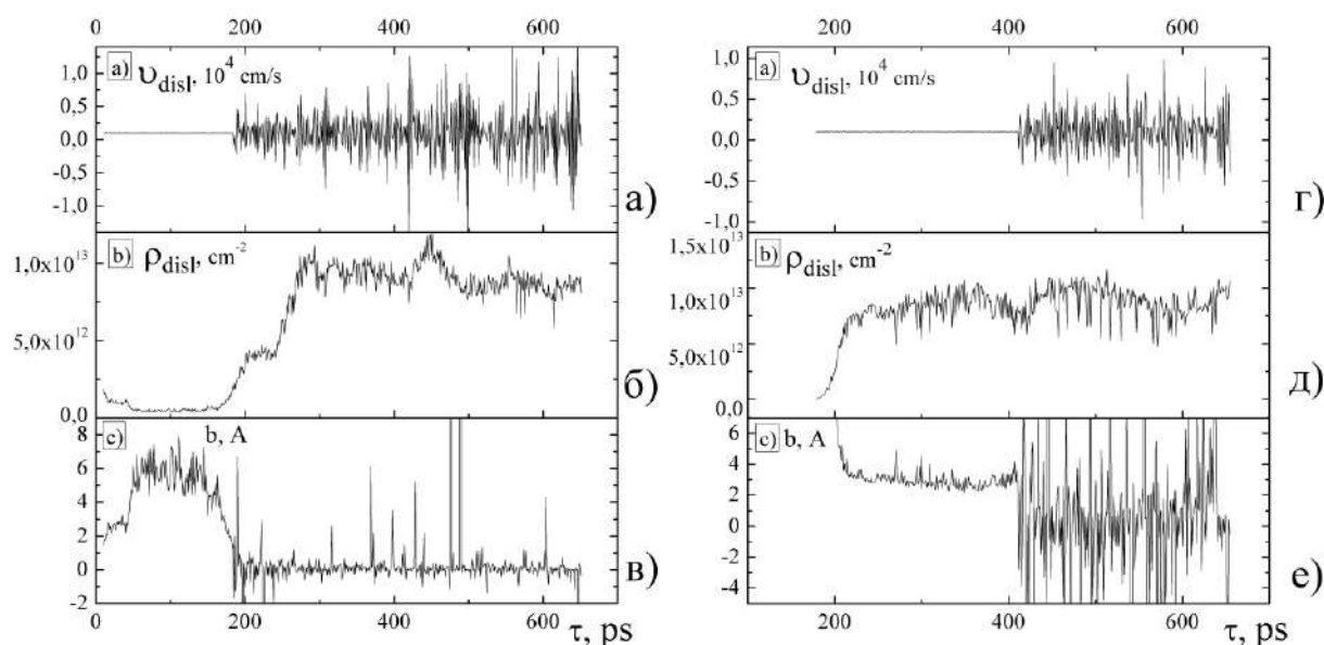
Рис. 2. а), б), в) – для [0001] –монокристалла магния с 5% вакансий, г), д), е) – для [10\bar{1}1] –монокристалла магния с 10% вакансий, а), г) – скорости дислокаций v_{disl} , б), д) – плотности дислокации \rho_m , в), е) – вектор Бюргерса b с учетом коэффициента \alpha , т.е. \alpha b
