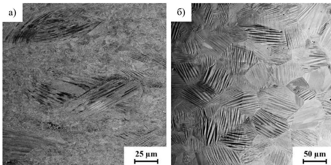
Рис. 2. Микроструктура сплава после отжига при 400°C (а) и 800°C (б) в течение 1 часа.
