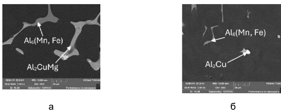
Рис. 2. Частицы в сплавах Al-Cu-Mn-Mg (Zr, Sc, Hf): № 2 (а), № 3 (б) (СЭМ)
