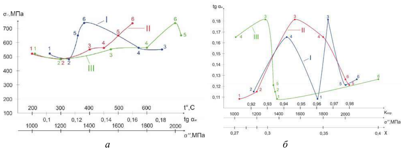
Рис. 3. а – Зависимости предела выносливости от: I – параметра сопротивления усталости; II – режима термоупрочнения; III – параметра микропластичности; б - Зависимости показателя сопротивления усталости от: I – коэффициента корреляции; II – параметра микропластичности; III – относительного коэффициента ограниченной выносливости
