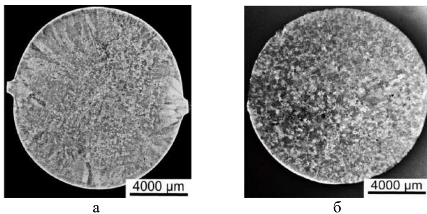
Рис. 1. Сравнительные результаты металлографических исследований макроструктуры поперечных сечений слитков сплава Al-2,5Fe (а) и композита на его основе (б)
