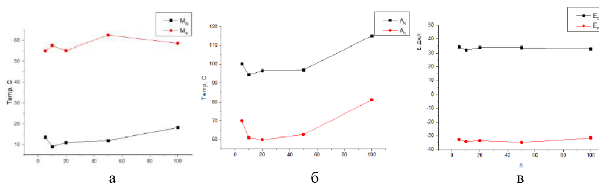
Рис. 1. Графики зависимости температур прямого (а), обратного (б) превращения и энергий превращения (в) от количества термоциклов в крупнозернистом состоянии
