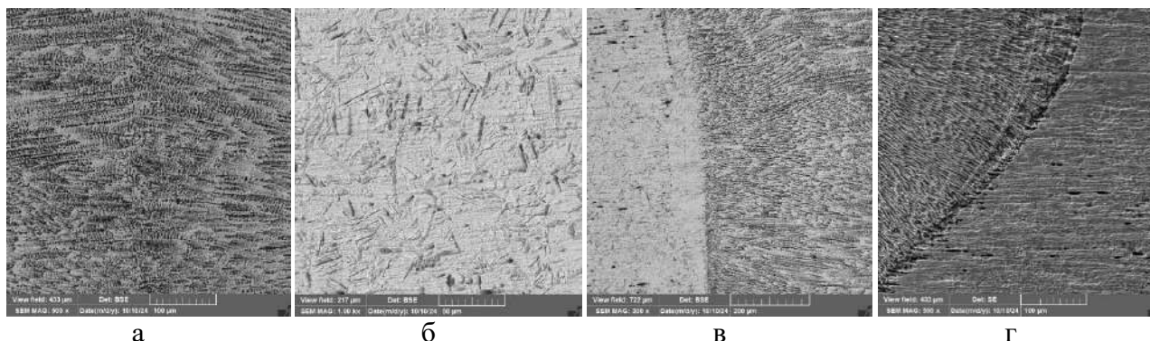
Рис. 2. Микроструктура различных участков сварного соединения из стали 12X18H10Т (а – сварной шов, б - основной материал, в,г - переходная зона)
