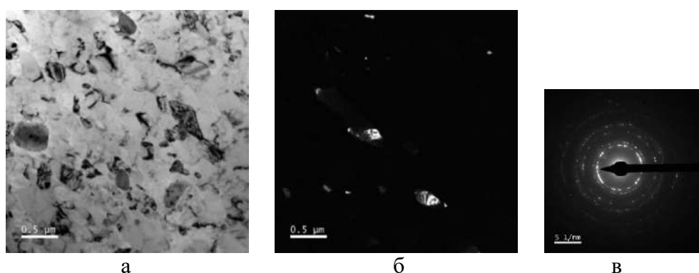
Рис. 2. Микроструктура композита: а – светлопольное изображение; б – темнопольное изображение в близких рефлексах (111)Al и (200)Al; в – кольцевая микроэлектронограмма
