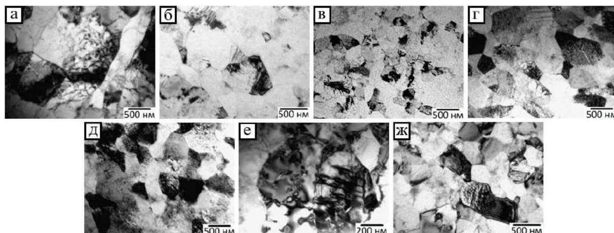
Рис. 2. Снимки микроструктуры сплава TiNi в УМЗ состоянии а) - УМЗ, б) - отжиг 250 °С 1 ч, в) отжиг 300 °С 1 ч, г) - отжиг 350 °С 1 ч, д) - отжиг 400 °С 1 ч, е) - отжиг 450 °С 1 ч, ж) - отжиг 500 °С 1 ч
