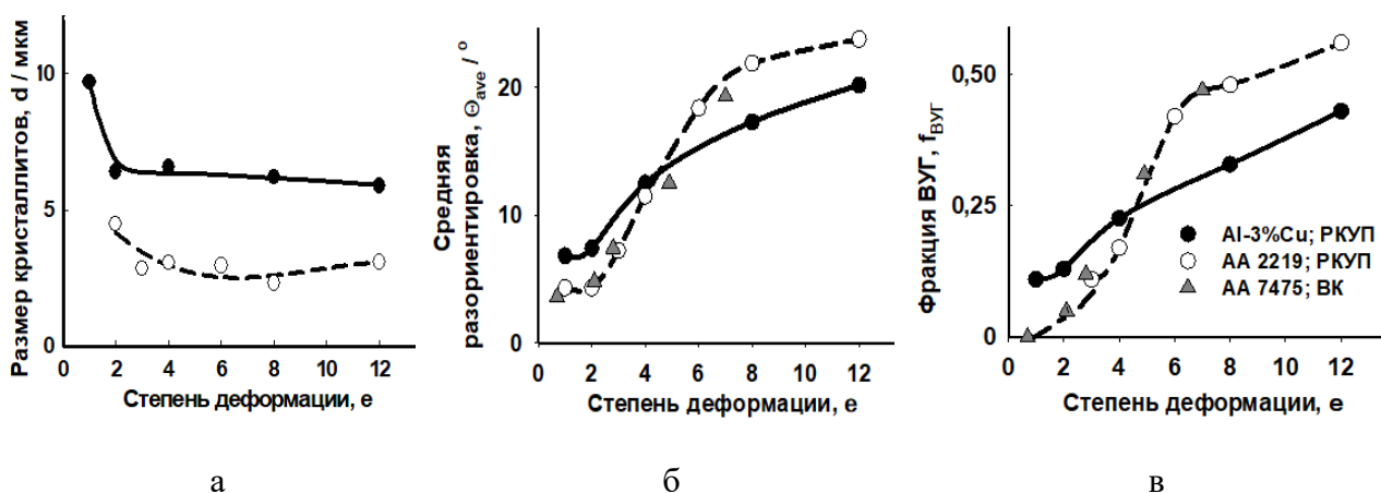
Рис. 2. Зависимости (а) размера новых кристаллитов, (б) средней разориентировки межкристаллитных границ и (в) доли ВУГ от степени деформации. ВК - всесторонняя ковка.
