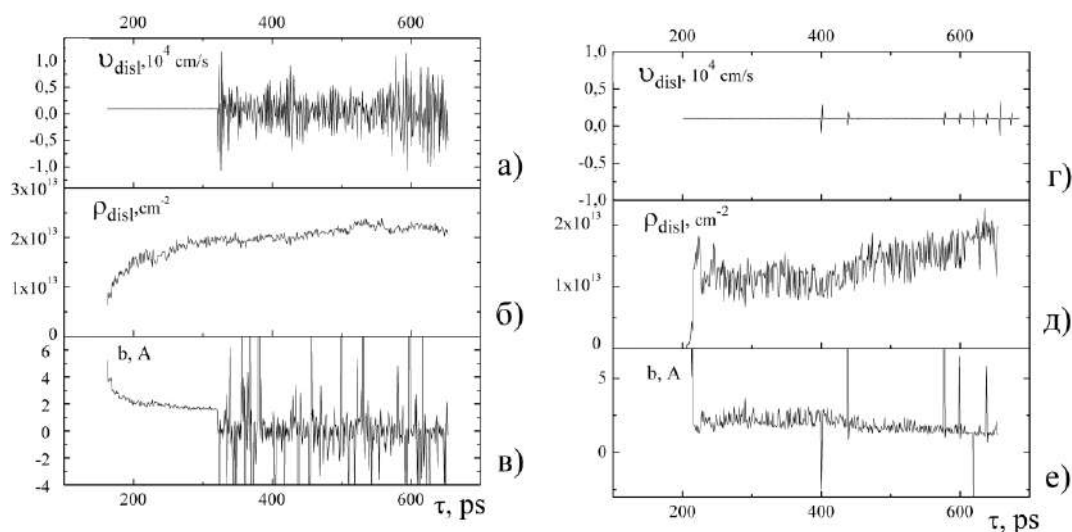
Рис. 1. а), б), в) – для [0001] – монокристалла магния, г), д), е) – для [10\bar{1}1] – монокристалла магния, а), г) – скорости дислокаций v_{disl} , б), д) – плотности дислокации \rho_m , в), е) – вектор Бюргерса b с учетом коэффициента \alpha , т.е. \alpha b
