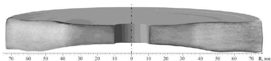
Рис. 3. Макроструктура модельного диска из сплава ЭП741НП после термообработки в градиентном температурном поле, деформации и упрочняющей термообработки.
