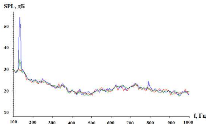
Рис. 5. Спектры излучения шума для угла установки авиационной конструкции 8^\circ при скорости потока V=12 м/с и воздействии на частоте 132 Гц, где: — исходный шум лопасти, — шум резонансного режима, — шум в режиме демпфирования
