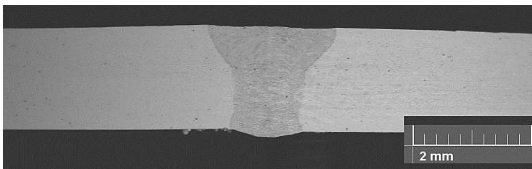
Рис. 1. Макроструктура сварного соединения нержавеющей стали 12X18H10Т
