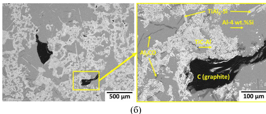
Рис. 2. Микроструктура и основные фазы СВС-композита: (а) - TiC-C-(Al-5%Cu) и (б) - TiC-C-(Al-5%Si)
