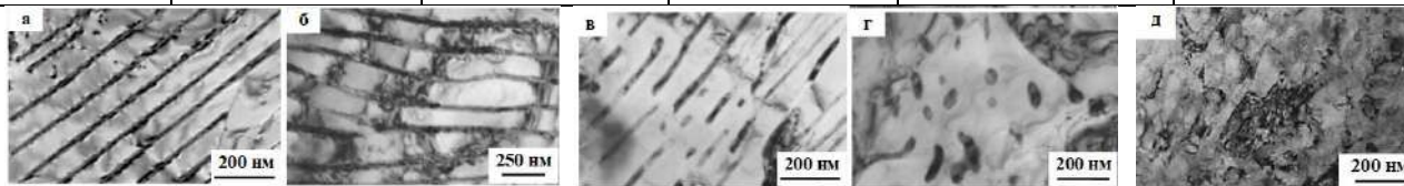
Рис. 1. Электронно-микроскопические изображения различных морфологических составляющих структуры заэвтектоидной стали Э90ХАФ [1]: а – пластинчатый не разрушенный перлит; б – фрагментированный не разрушенный пластинчатый перлит; в – разрушенный пластинчатый перлит; г – глобулярный перлит; д – субзеренная структура
