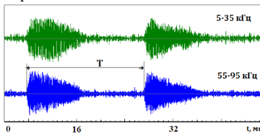
Рис. 2. Пример записей сигналов АЭ в 2х диапазонах частот при подаче 200 лазерных импульсов в лунку керамической пластины Al_2O_3 (Т – период подачи 200 импульсов)
