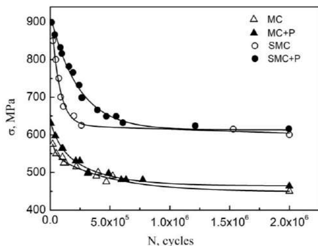
Рис. 1. Зависимость напряжения от количества циклов N до разрушения при усталостных испытаниях сплава ВТ1-0 в МК и СМК состояниях, а также после их обработки высоким гидростатическим давлением (+P). [1]
