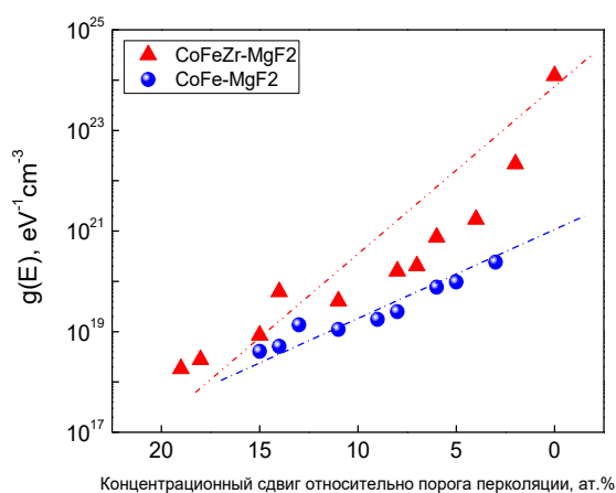
Рис. 1. Зависимость плотности электронных состояний на уровне Ферми в композитах (CoFe) x (MgF 2 ) 100-x и (CoFeZr) x (MgF 2 ) 100-x от концентрационного положения образца относительно порога перколяции
