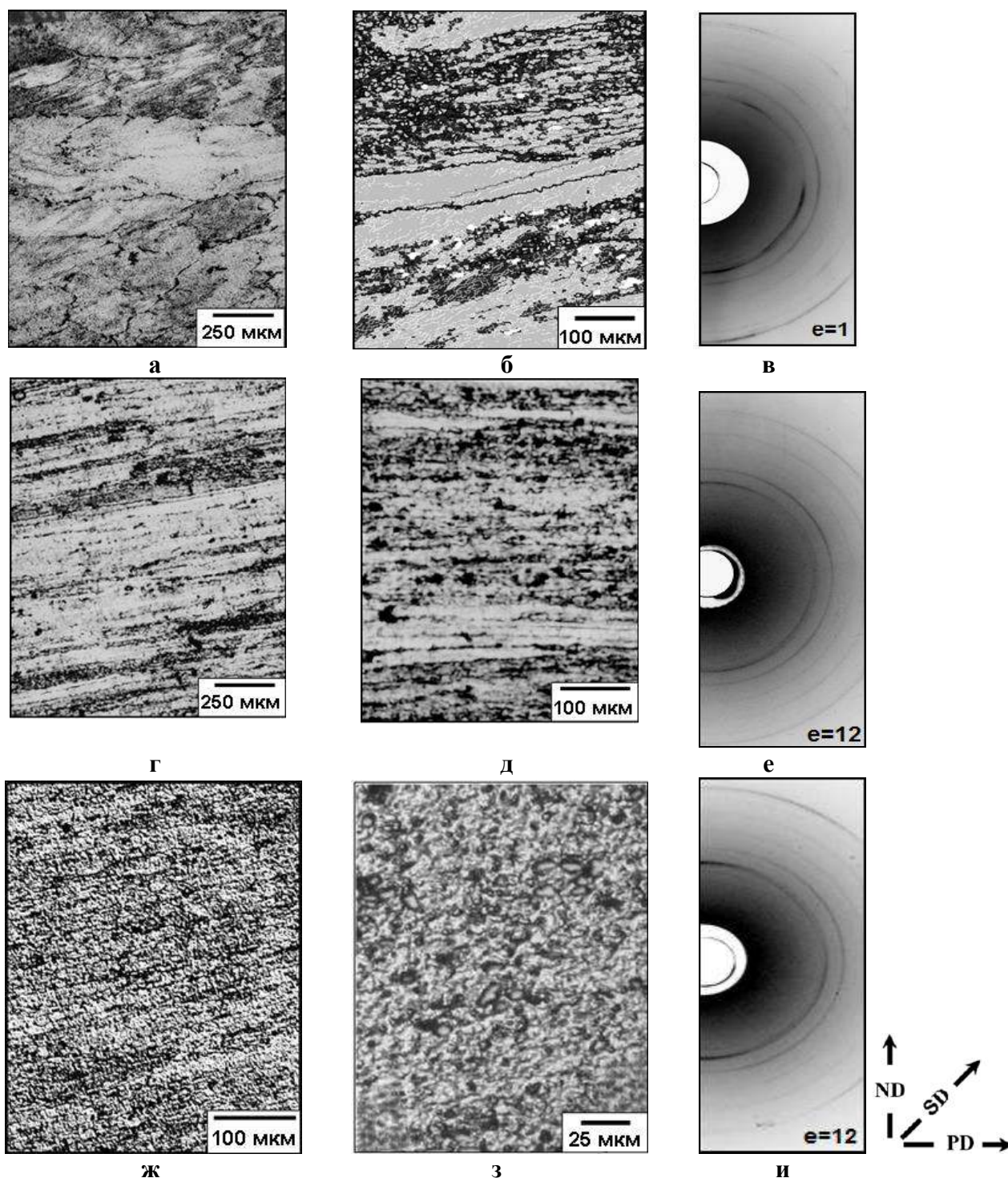
Рис. 1. Микроструктура сплавов Al-3%Cu и AA2219 после РКУП при 300°C. (а-в) Al-3%Cu, e=1 , (г) Al-3%Cu, e=4 , (д, е) Al-3%Cu, e=12 , (ж-и) AA2219, e=12 . (а, г, д, ж, з) оптическая микроскопия, (б) EBSD анализ, (в, е, и) рентгеновские дифракционные картины.
