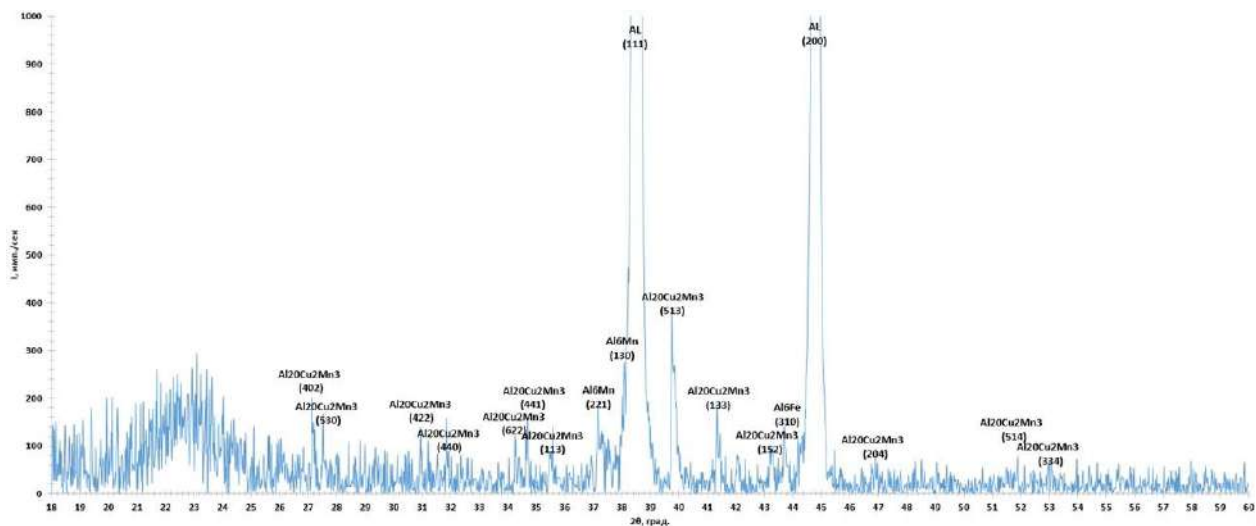
Рис. 3. Участок дифрактограммы состава №4
