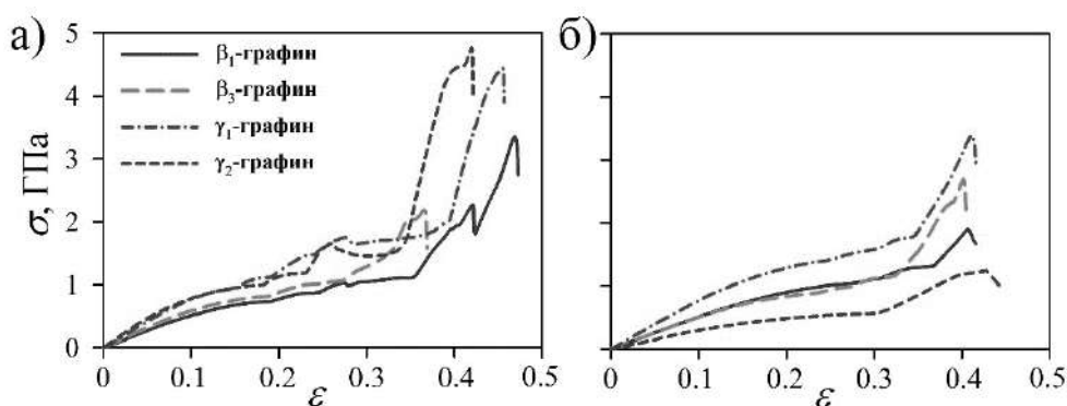
Рис. 2. Кривые «напряжение-деформация» для четырех графитов ( \beta_1 -, \beta_3 -, \gamma_1 - и \gamma_2 -) при растяжении в направлениях кресло(A) и зигзаг (B)
