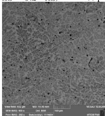
Рис. 1. Микроструктура образца сплава Ni 37 Co 13 Mn 35 Ti 15 , полученная в режиме композиционного контраста в SEM.
