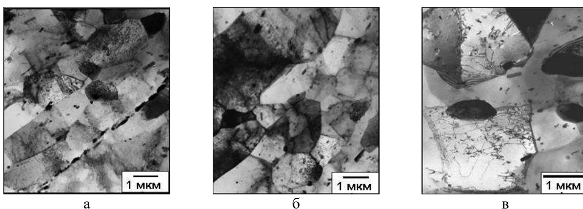
Рис. 3. ПЭМ изображения микроструктуры, развившейся в сплаве AA2219 в результате РКУП при 300°C (а) e=3 ; (б) e=8 и (в) e=12 . (в) представлено при большем увеличении.
