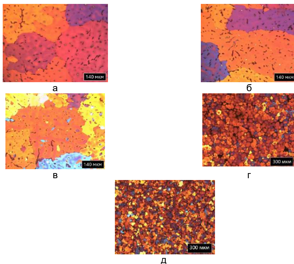
Рис. 1. Микроструктура сплавов Al-Cu-Mn-Mg (Zr, Sc, Hf): № 1 (а), № 2 (б), № 3 (в), № 4 (г), № 5 (д)
