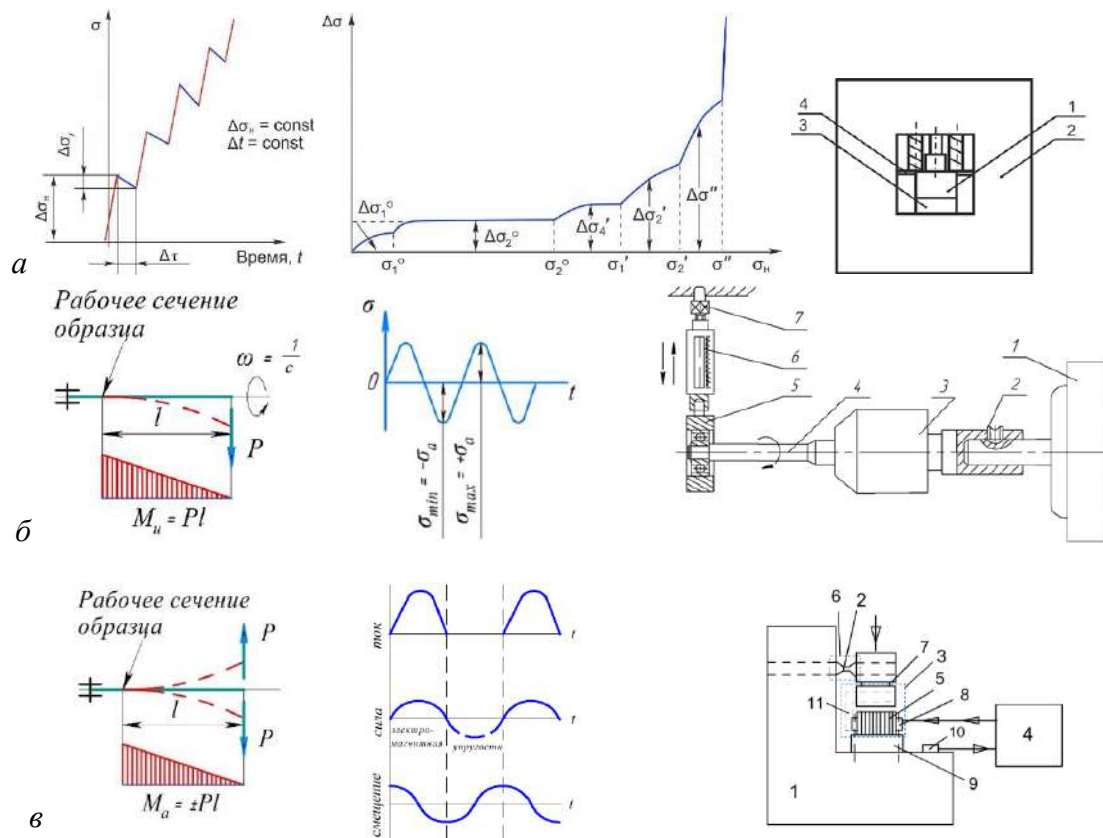
Рис. 1. Изображения: а – схемы деформирующего устройства для испытаний на исследование особенностей микропластической деформации, релаксации напряжений, ступени нагружения и зависимости \Delta\sigma ( \Delta\sigma_n ), отражающие поэтапное развитие пластической деформации ограниченных критическими напряжениями \Delta\sigma^0, \sigma', \sigma'' , которые характеризуют способность сплавов сопротивляться малым пластическим деформациям; б – схемы установки для испытаний на усталость при консольном изгибе с вращением, распределения напряжений в цикле и моментов сил; в – схемы установки для испытаний на частотную стабильность, распределения нагрузки при консольном циклическом поперечном изгибе плоского образца и согласования импульсов тока, электромагнитной силы и силы упругости с перемещением консоли исследуемого образца в этой установке
