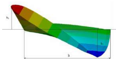
Рис. 2. Схема расчета угла закручивания авиационной композитной конструкции с изменяемой геометрией
