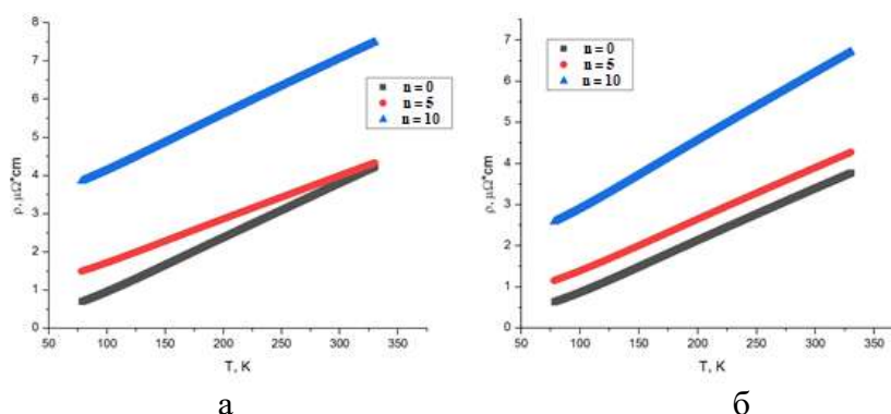
Рис. 3. Температурная зависимость удельного электросопротивления матричного сплава (а) и композита (б) после кручения в зависимости от числа оборотов
