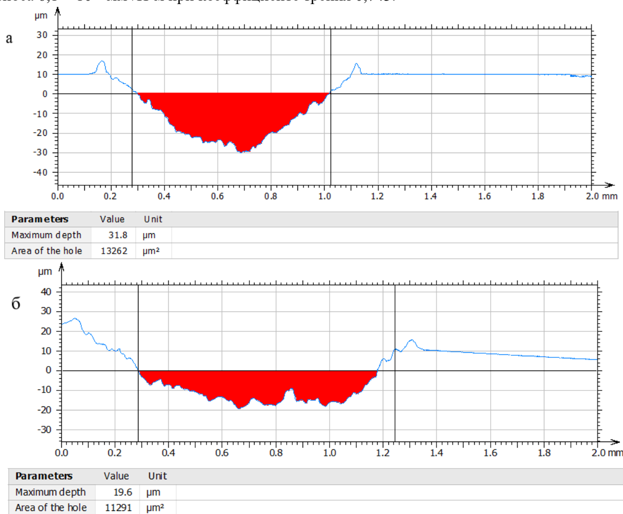
Рис. 1. Профили дорожки трения образцов высокоэнтропийных сплавов \text{Co}_{20}\text{Cr}_{20}\text{Fe}_{20}\text{Mn}_{20}\text{Ni}_{20} (а) и \text{Co}_{25}\text{Cr}_{25}\text{Fe}_{15}\text{Mn}_{15}\text{Ni}_{20} (б)
