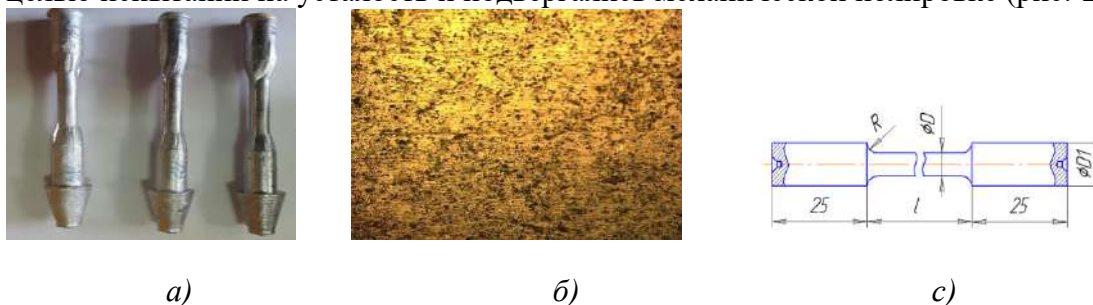
Рис. 1. Изображения: а-литые цилиндрические образцы, полученные методом литья в стальную форму; б-микроструктура сплава (х 100); в-эскиз цилиндрического образца для усталостных испытаний: D=7,5\text{мм} ; D1=12\text{мм} ; R=10\text{мм} ; l=90\text{мм} .
