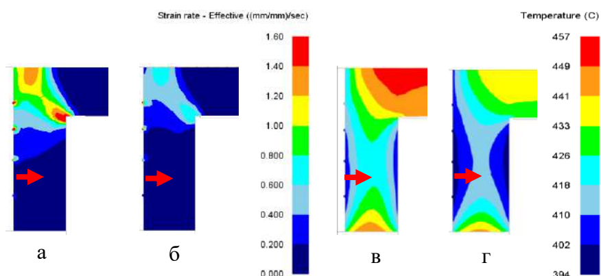
Рис. 2. Распределение на заключительной стадии процесса: скорости деформации для первого (а) и второго (б) варианта прессования, температурного поля для первого (в) и второго (г) варианта прессования, стрелка показывает направление движения пресс-штемпеля
