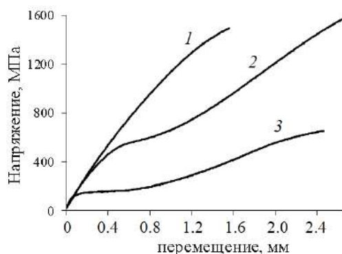
Рис. 2. Кривые напряжение-перемещение в состояниях 1, 2, 3, указанных в табл. 1.
