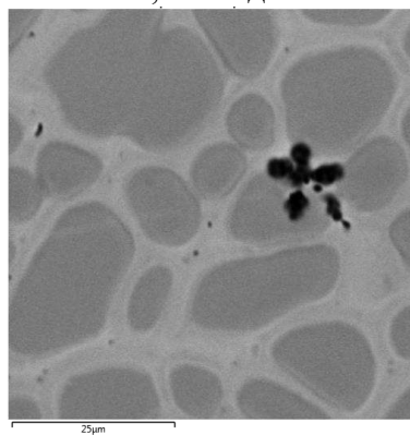
Рис. 1. Микроструктура образца сплава Ni 37 Co 13 Mn 35 Ti 15 , полученная в режиме композиционного контраста в SEM.
