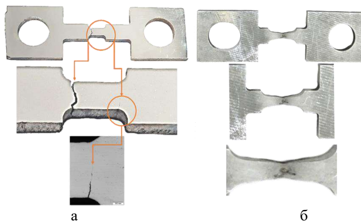
Рис. 1 (а) – типичная локализация магистральной трещины в образцах типа ДСП после испытаний на термическую усталость; (б) – образовавшаяся шейка и трещина в образце типа ДСП при испытаниях с многократным повторением полуцикла охлаждения
