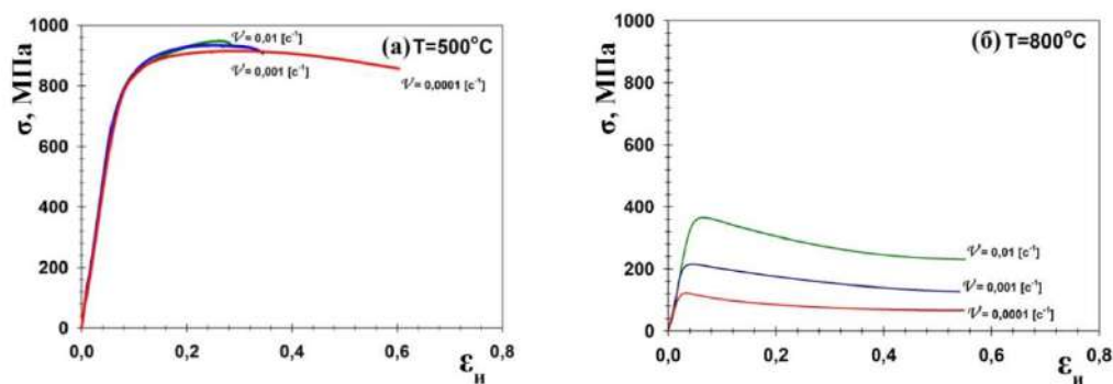
Рис. 1. Истинные диаграммы сжатия исходного состояния сплава TA15
