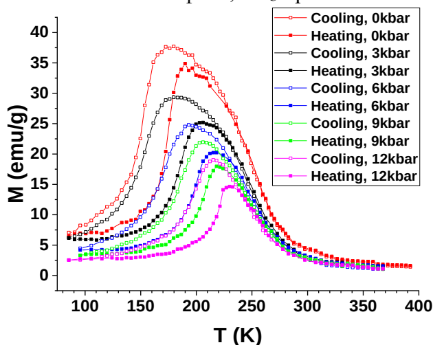
Рис. 2. Температурные зависимости намагниченности в поле 0.155 Тл (нагрев и охлаждение) для быстрозакалённых лент сплава \text{Ni}_{37}\text{Co}_{13}\text{Mn}_{35}\text{Ti}_{15} под внешним гидростатическим давлением от 0 до 12 кбар.
