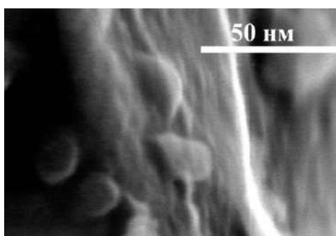
Рис. 2. Гидрированный графен
