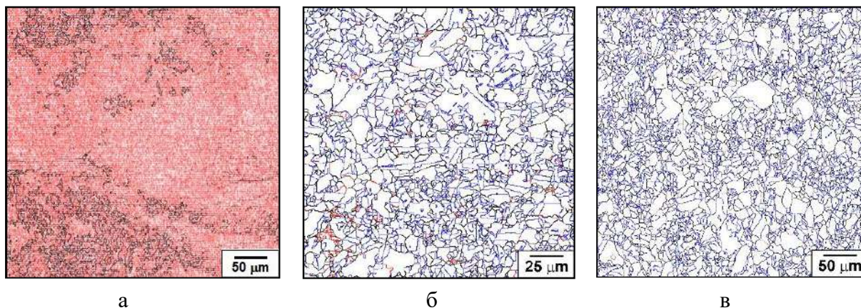
Рис. 1. EBSD карты межкристаллитных границ никеля после КП (а) и последующей ЭИО с K_j = 1.1 (б) и 1.6×10 4 А 2 с/мм 4 (в). Красные, черные и синие линии - мало-, высокоугловые и двойниковые ( \Sigma 3 + \Sigma 9 ) границы соответственно.
