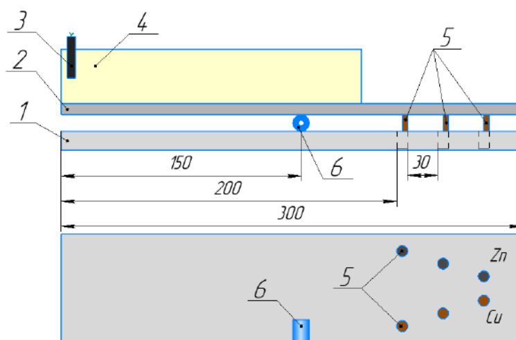
Рис. 1. Схема измерения яркостной температуры и установки термолловушек в зазоре: 1-основная пластина, 2-метаемая пластина, 3-детонатор, 4-взрывчатое вещество, 5-термолловушки; 6-оптический датчик для измерения яркостной температуры
