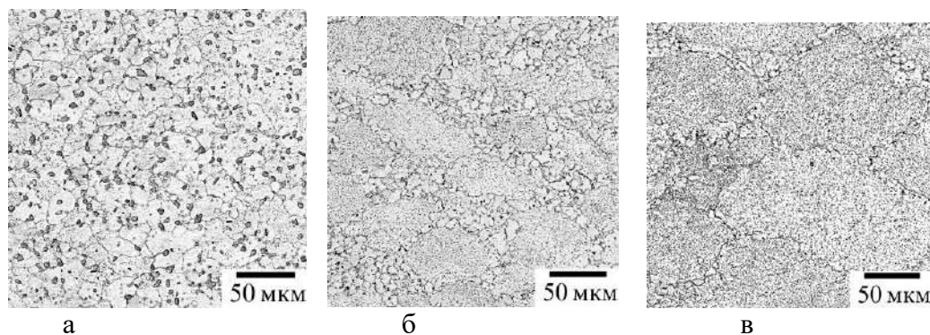
Рис. 4. Микроструктура модельного диска в ступице (а) и в ободе на R=50 мм (б) и на R=70 мм (в)
