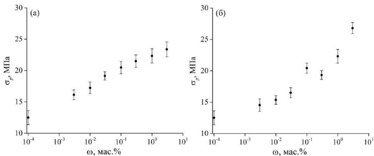
Рис. 1. Зависимости прочности на сжатие \sigma_p от массовой доли \omega наполнителя для ЛК с НЧ (а) и ПВС (б)
