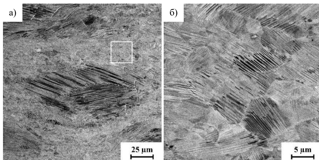
Рис. 1. Микроструктура сплава после всесторонней изотермическойковки (а), прослойка мелкозернистой структуры (б).
